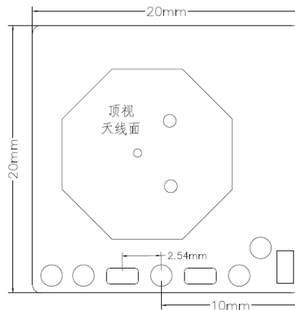
图 4.2 RA5U11-B 模块尺寸图 (引脚兼容2.54mm与2.0mm排针)
