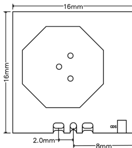
图 4.2 RA5U16-B 模块尺寸图 (引脚兼容2.54mm与2.0mm排针, 并且邮票口可以贴片安装)
