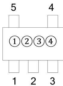
SOT23-5
