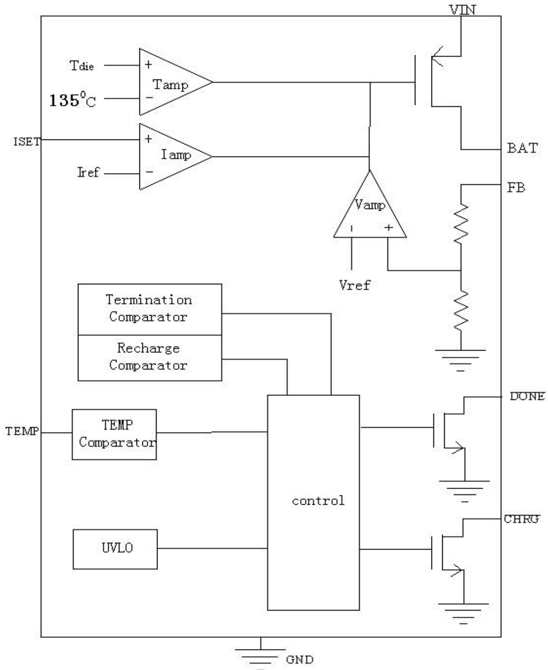
图 3 功能框图
